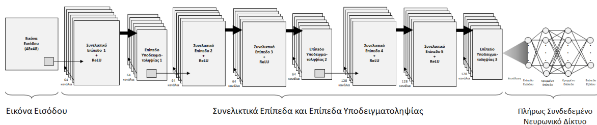
Σχήμα 10. Η αρχιτεκτονική του Συνελικτικού Νευρωνικού Δικτύου για την αναγνώριση συναισθημάτων
